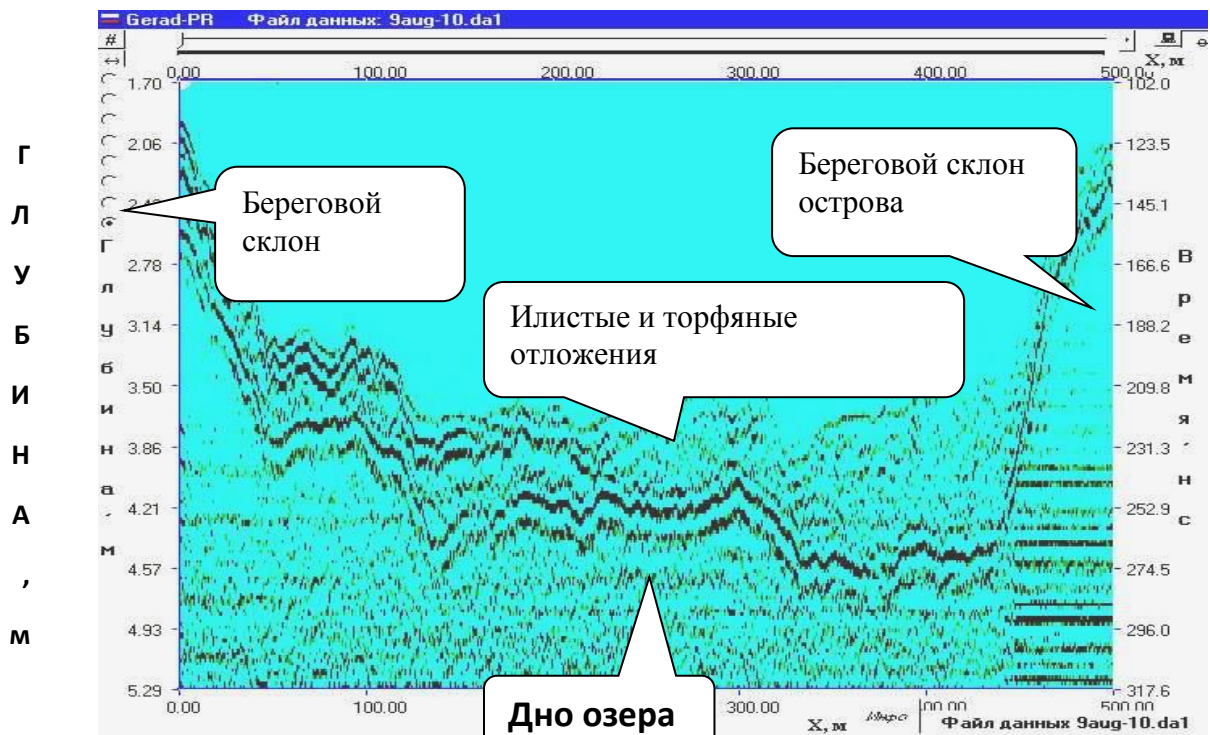
Рис.3. Результаты профилирования дна озера большое георадаром Герад 3 (200 МГц).
