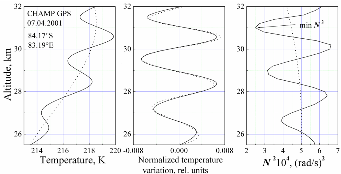
Рис. 1. Волновые возмущения, наблюдаемые из вертикального профиля температуры (7 апреля 2001 года) радиозатменной миссии ШАМР в полярной атмосфере над Антарктикой. Параметры внутренней волны: \lambda_z=2.2 км; \lambda_h=1230 км; E=70 Дж/кг; p=E_k/E_p=30 ; E_p=2.3 Дж/кг; f/\omega=0.97 ; T''=2\pi/\omega=11.6 час; a_e=0.41 ; |u'|=11.8 м/с; |v'|=11.5 м/с
